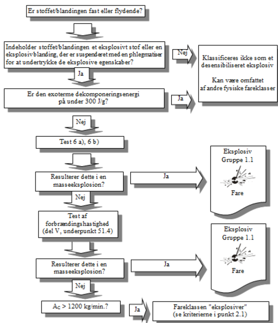
Figur 2.17.1. Desensibiliserede eksplosiver
