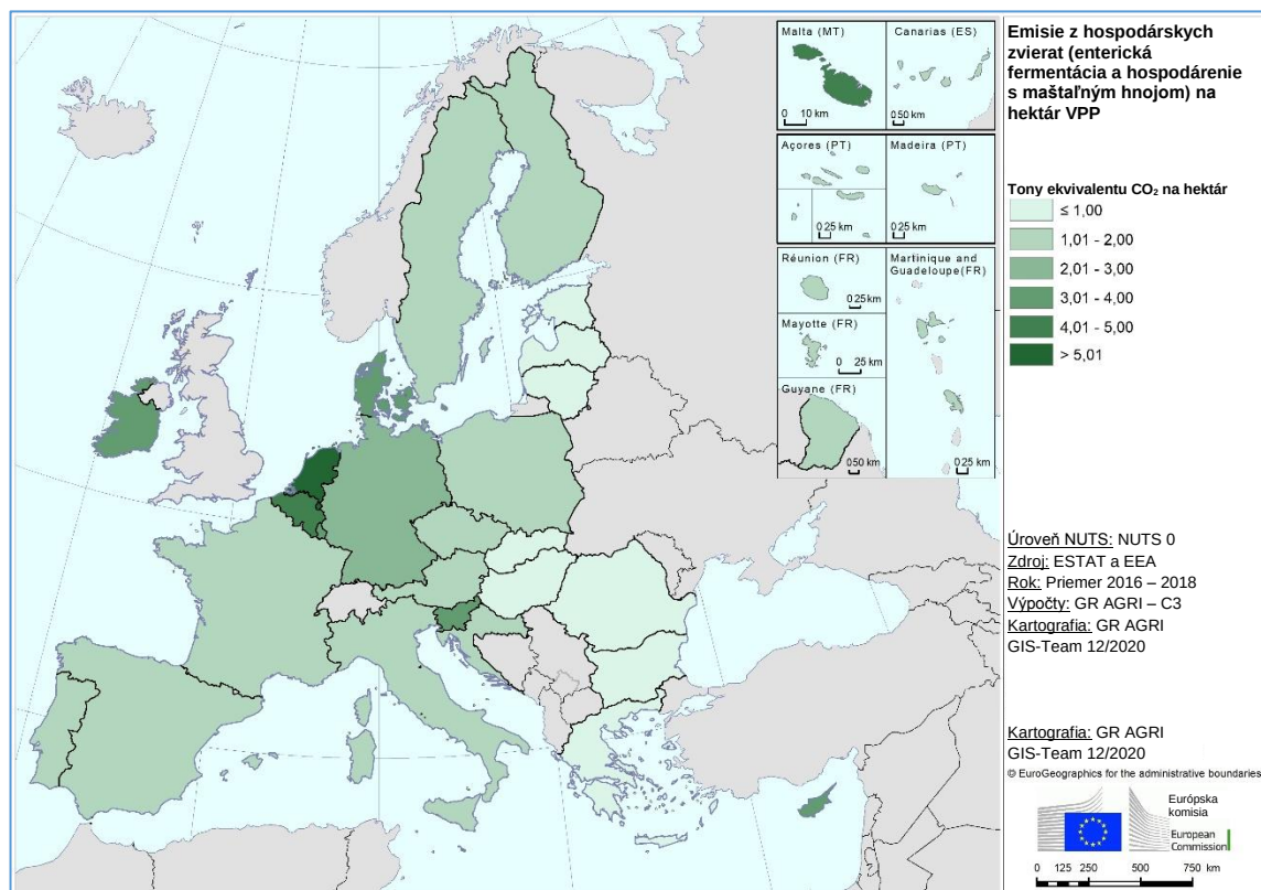
Mapa 1: Emisie skleníkových plynov z hospodárskych zvierat a enterická fermentácia za výrobné faktory v EÚ
