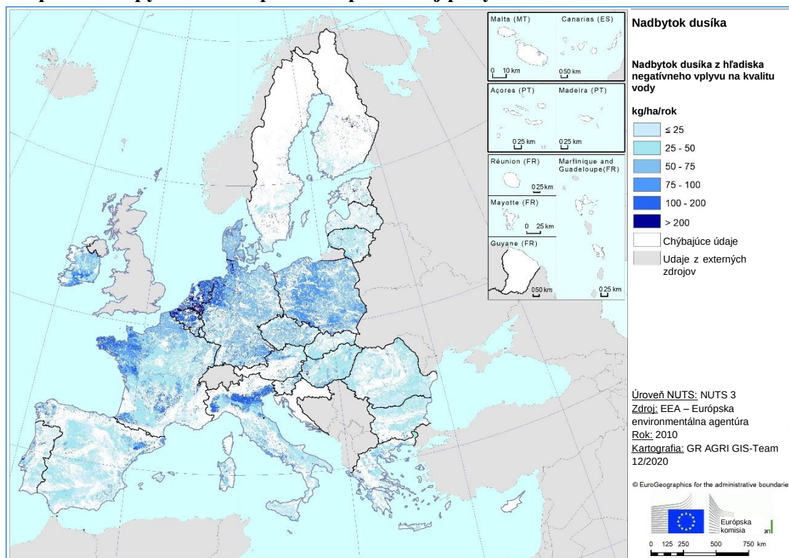
Mapa 2: Vstupy dusíka do poľnohospodárskej pôdy v EÚ
