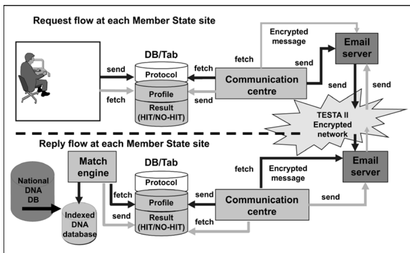
Figur 3: Tillämpningens arbetsflöde vid staternas anläggningar, översikt
