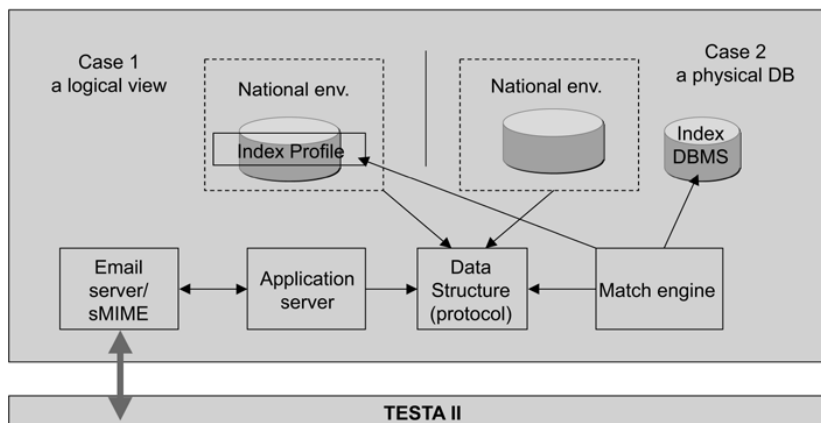
Figur 2: Översikt av tillämpningstopologin
