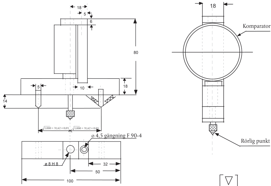
Figur 3: sfärometer
