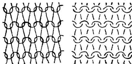
Figur 1 Enkeljersey (slätstickning)
