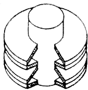
Staplade tallriksfjädrar (i genomskärning)
