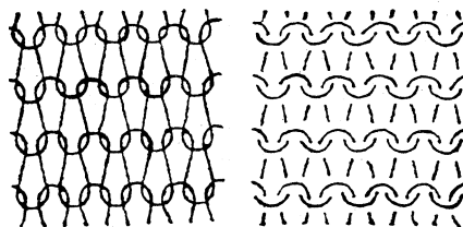
Figur 1 Enkeljersey (slätstickning)
