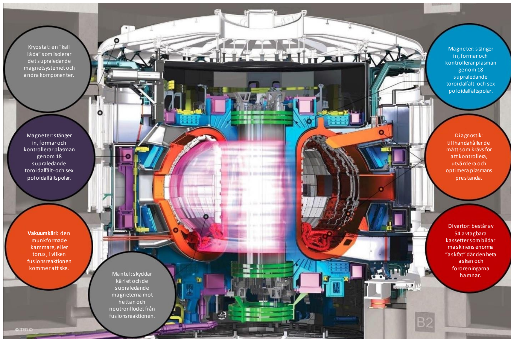
Figur 1: ITER-tokamaken i genomskärning, med korta förklaringar av huvudsystemens funktioner. Källa: 2016 års statusrapport för det gemensamma företaget. Upphovsrätt: Iter-organisationen
