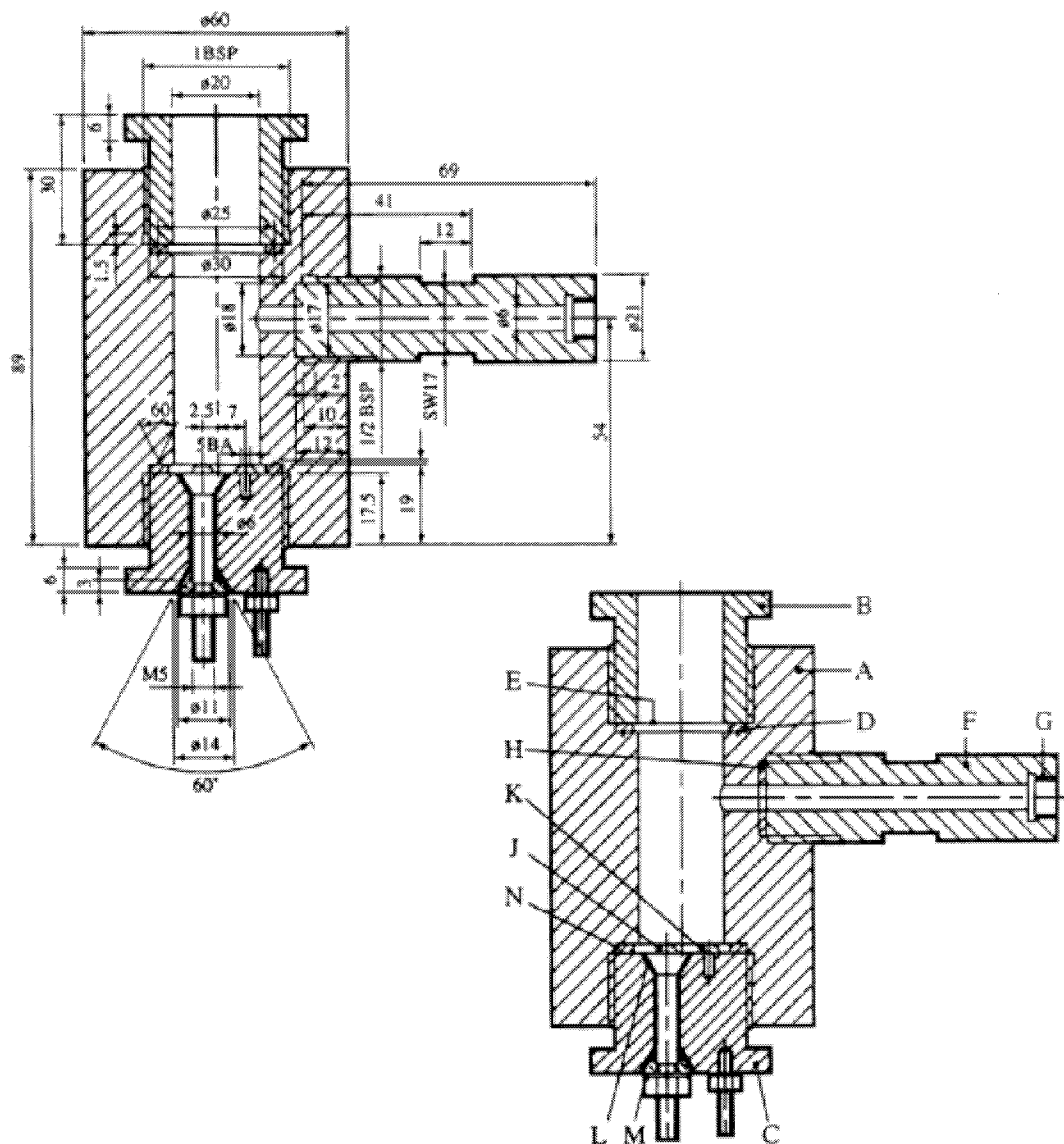
Tryckkärl
