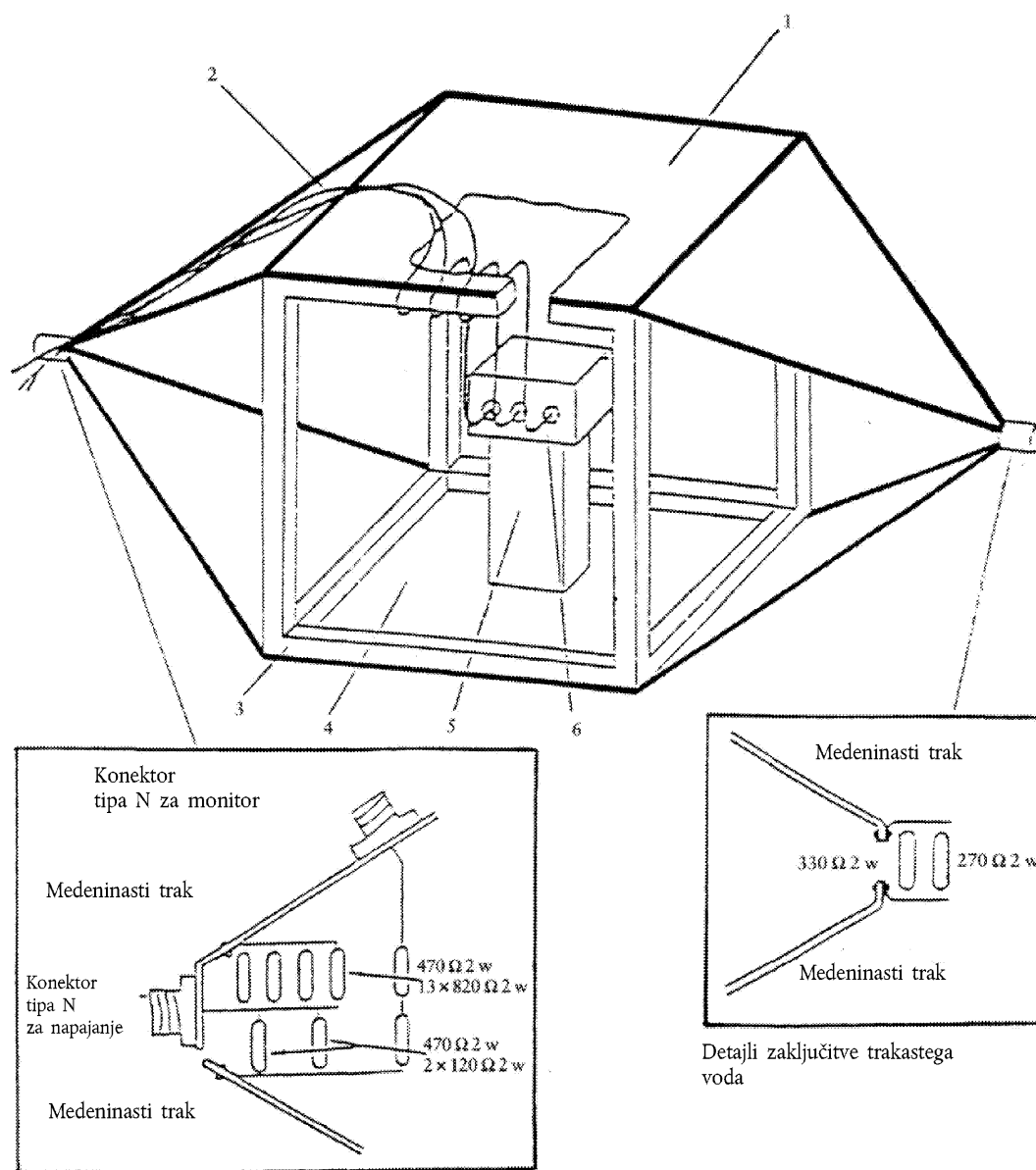
Detajli napajalnega dela t rakastega voda
