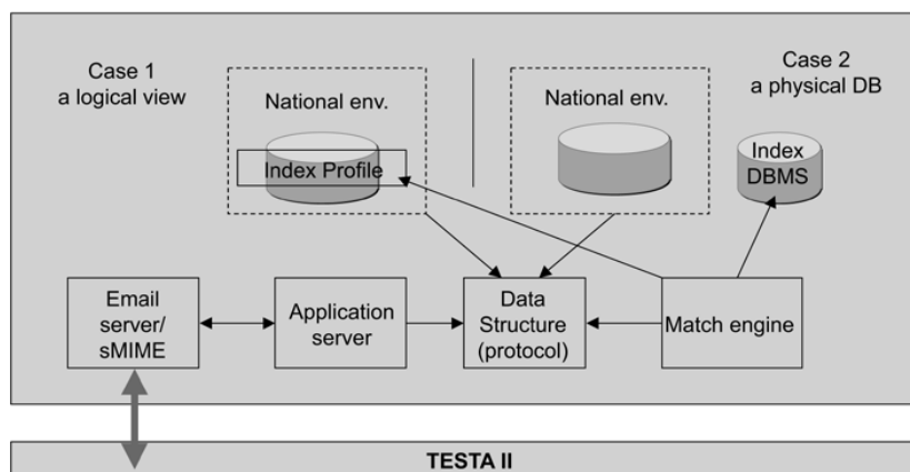
Obrázok 2: Prehľad aplikačnej topológie
