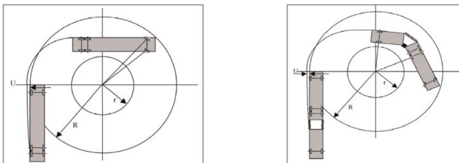
Obrázok 2a: vybočenie zadnej časti vozidla (nekľbové vozidlá) Obrázok 2b: vybočenie zadnej časti vozidla (kľbové vozidlá)
