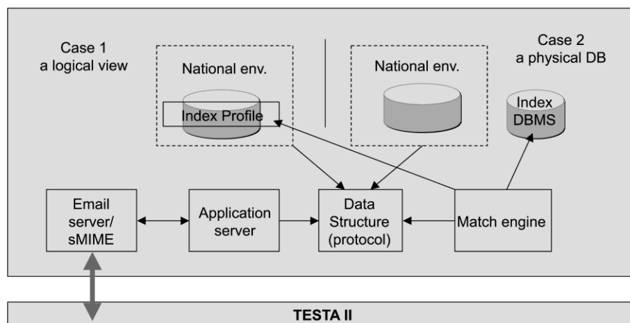
Obrázok 2: Prehľad aplikačnej topológie
