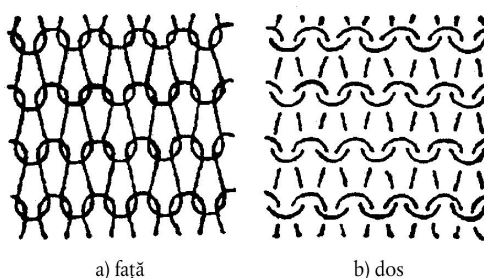
Figura 1 Tricostat simplu (tricostat plat)
