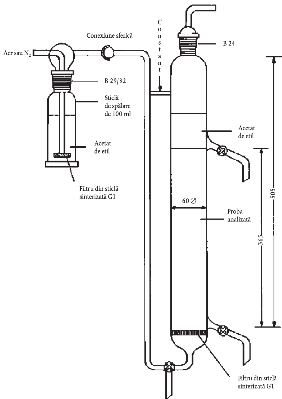
Figura 5 Aparat de separare cu gaze (dimensiunile în milimetri)
