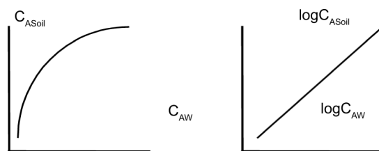
Figura 2 Reprezentarea grafică a ecuației Freundlich, normală și linearizată
