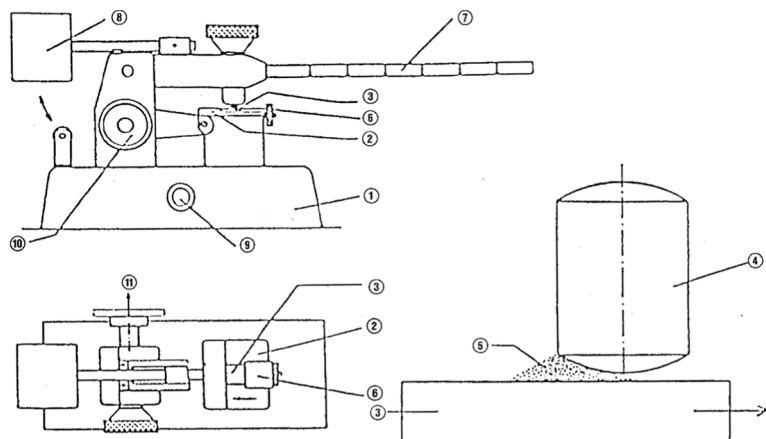
Figura 5b Poziția de pornire a știftului pe probă
