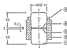
Figura 4d Dispozitivul de șoc pentru substanțele lichide
