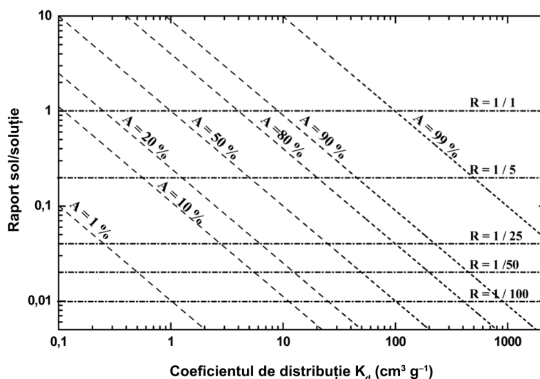
Figura 1 Relația dintre raporturile sol/soluție și K_d la diferite procente de substanță testată adsorbită
