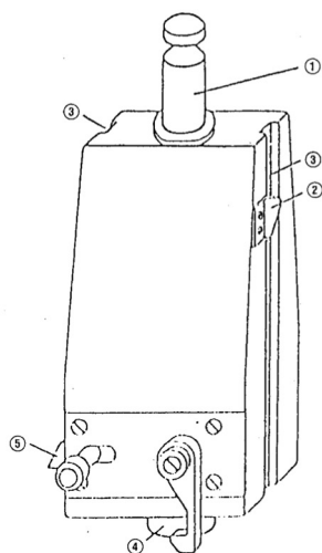
Figura 4e Ciocanul (masa de 5 kg în cădere)
