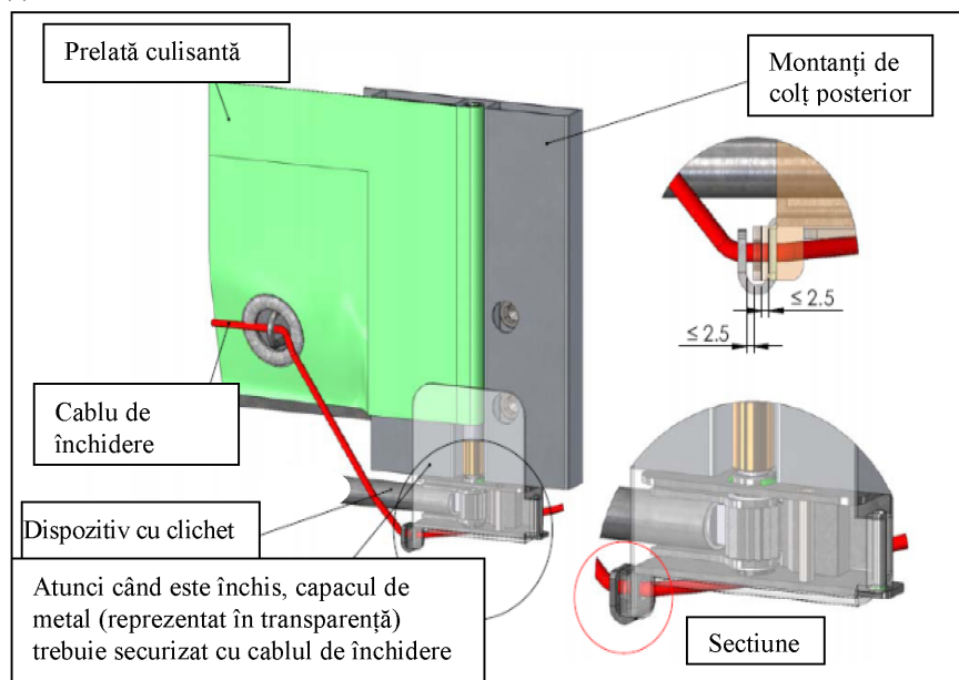
(b) Securizarea dispozitivului de întindere cu reductor
