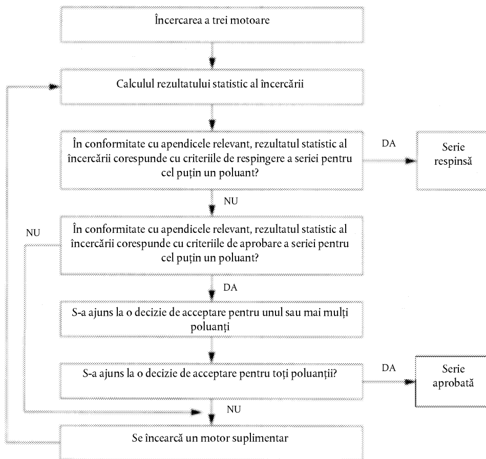
Figura 2.1 Schema logică a încercării privind conformitatea producției
