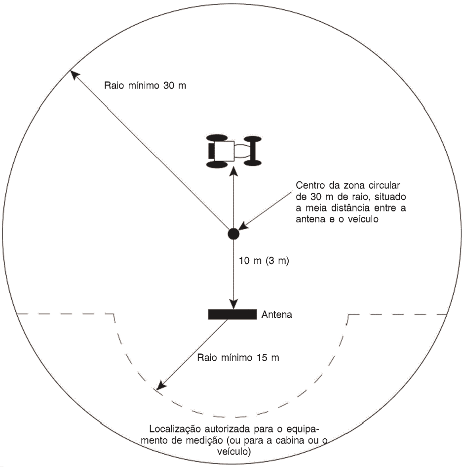
Figura 1 Zona de ensaio do trator (Superfície horizontal desimpedida isenta de reflexão eletromagnética)
