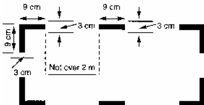
Oznakowanie miejsc awaryjnego cięcia kadłuba
