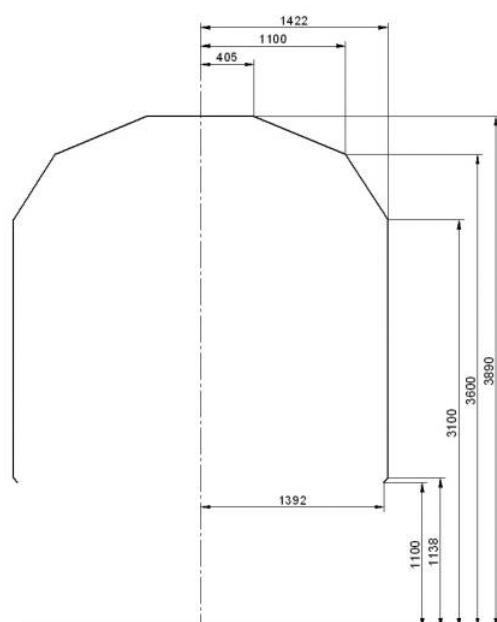
C.3 Profil górnego sektora UK1[A] powyżej 1 100 mm nad płaszczyzną toru
