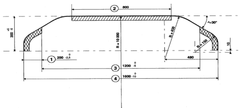
Profil ślizgacza pantografu
