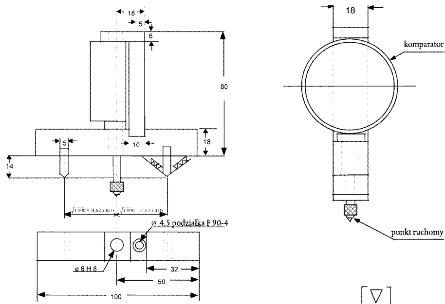
Rysunek 3. Sferometr
