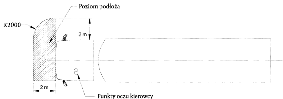
Rys. 11. Pole widzenia w przypadku lustra klasy VI
