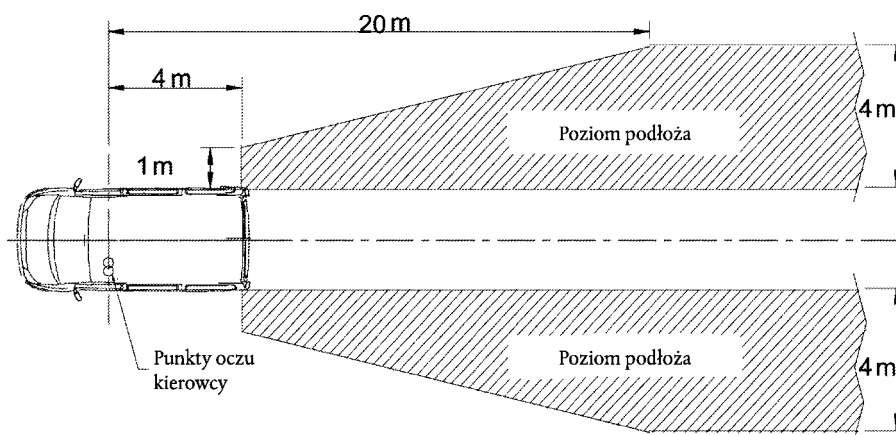
Rysunek 8. Pole widzenia w przypadku lustra klasy III
