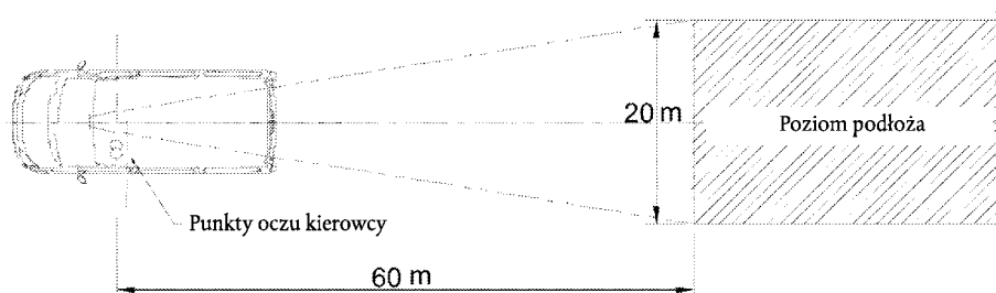
Rysunek 6. Pole widzenia w przypadku lustra klasy I
