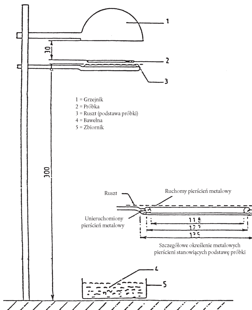
Rysunek 1 (Wymiary w milimetrach)
