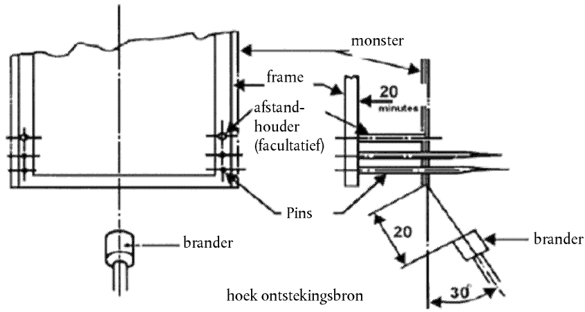
Figuur 3 Gasbrander (afmetingen in mm)
