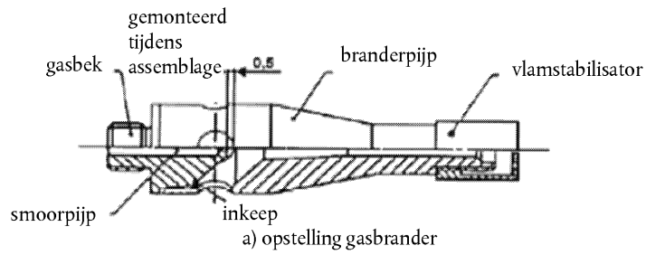
Figuur 3 Gasbrander (afmetingen in mm)
