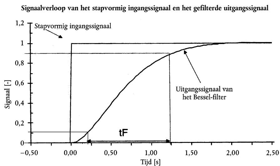
Figuur a toont het verloop van het stapvormige ingangssignaal en het uitgangssignaal van het Bessel-filter en de responsietijd ( t_F ) van het Bessel-filter.
