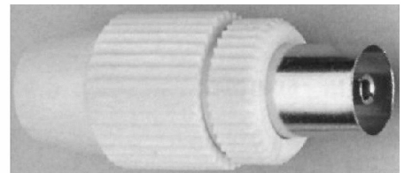
Afbeelding 2 Coaxiale contrastekker
