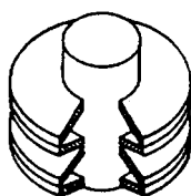
Gelaagde schotelveer (opengewerkt)
