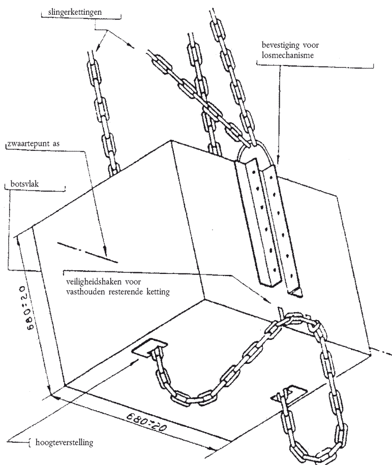
Figuur 3.1 Slingerblok en de draagkettingen of -kabels ervan (afmetingen in mm)
