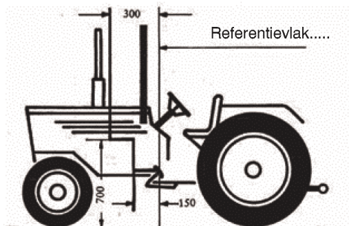
Figuur 1 (afmetingen in mm)
