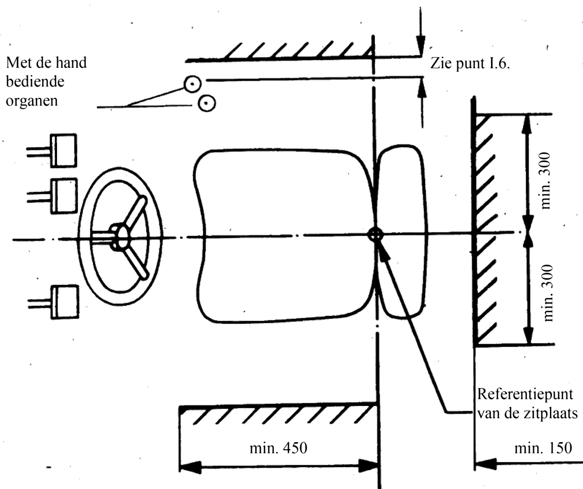
Figuur 3 (Afmetingen in millimeter)
