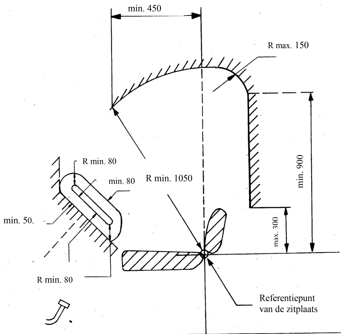
Figuur 2 (Afmetingen in millimeter)
