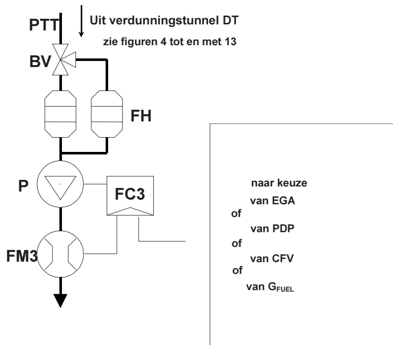
Deeltjesbemonsteringssysteem
