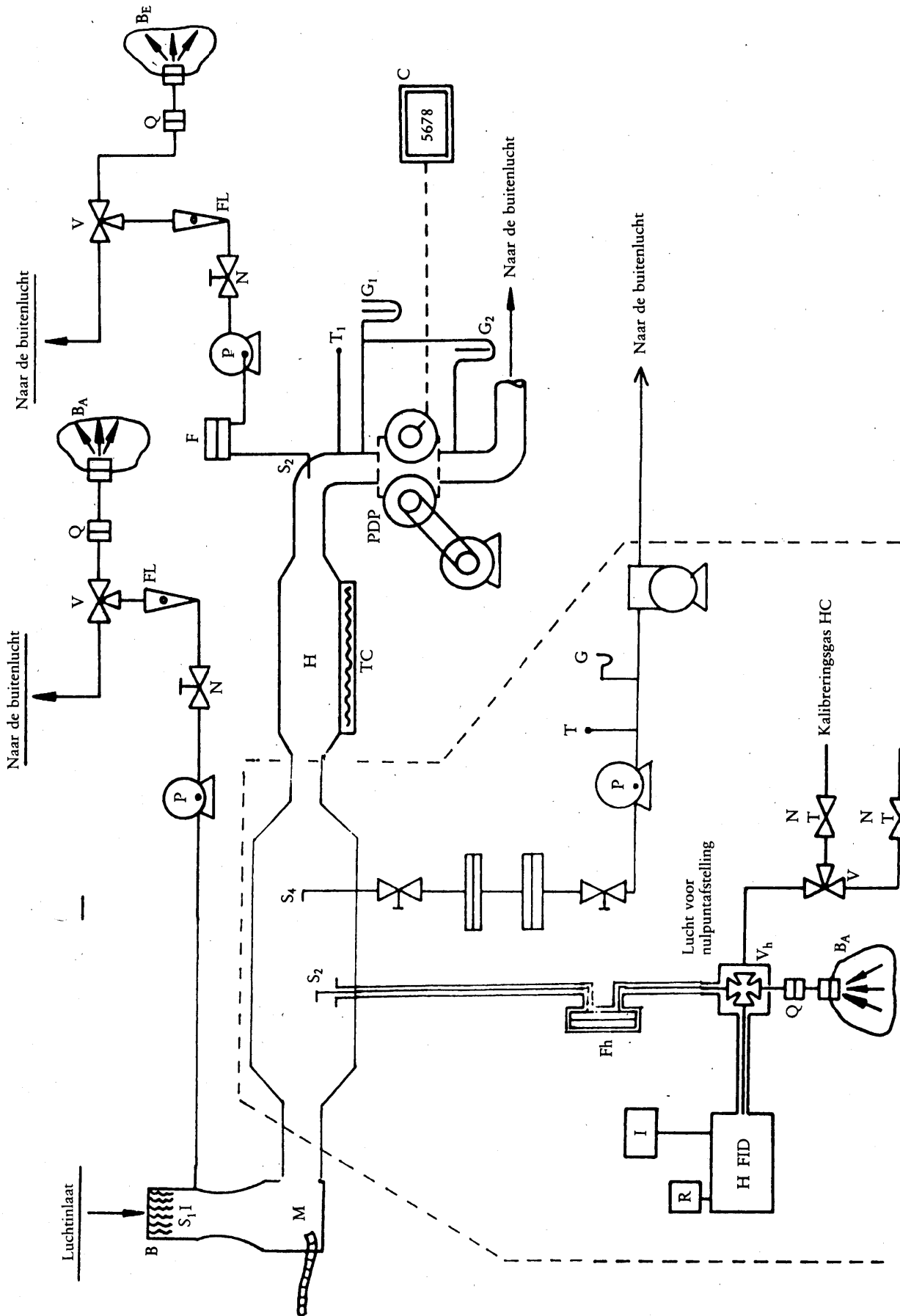
Schema van een bemoneeringsysteem met constant volume met verdringingspomp (PDP-CVS)
