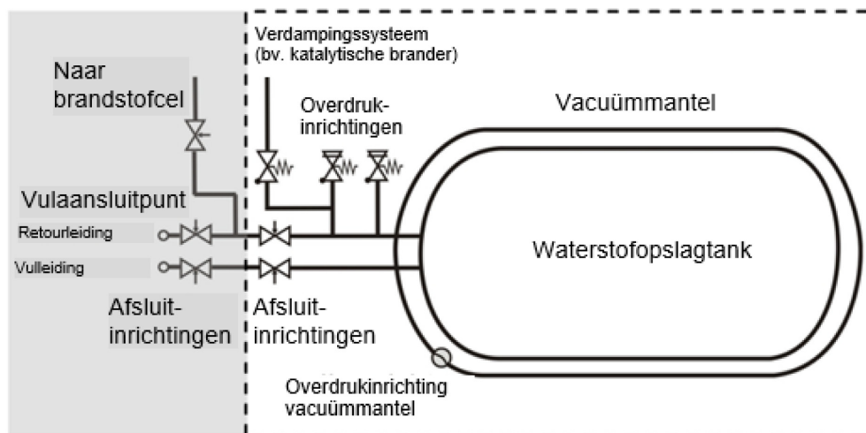
Typisch opslagsysteem voor vloeibare waterstof
