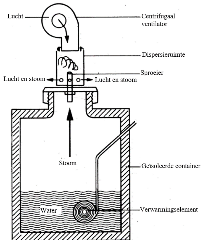
Schema stoomgenerator
