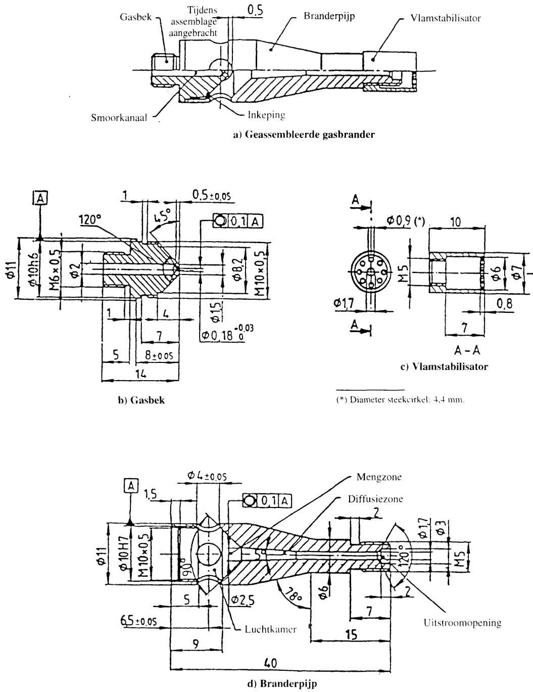
Figuur 3 Gasbrander (Afmetingen in mm)
