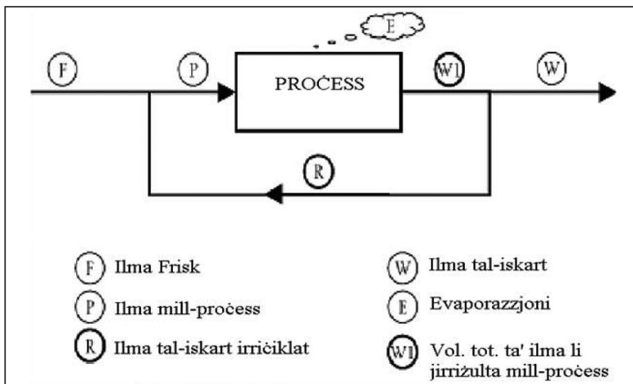
Figura A1: L-iskema tal-fluss tal-ilma li għandha tintuza għall-kalkolu tal-Proporzjon tar-Riċiklaġġ tal-Ilma (1)
