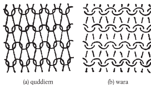
Figura 1 Ġersi singlu (hjata sempliċi)
