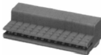
Figura 8 Konnetter b'ġenb wiehed għal konnessjoni diretta għal bord ta' ċirkuwit
