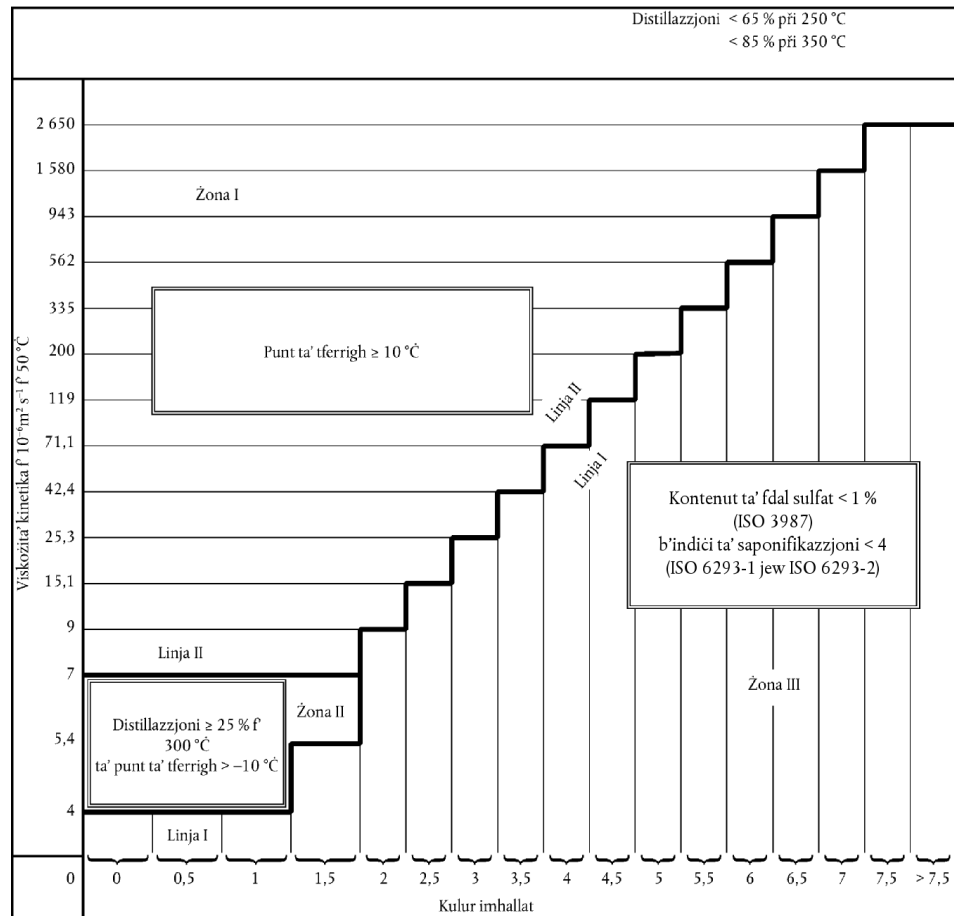
Karatteristiċi ta' żjut karburanti
