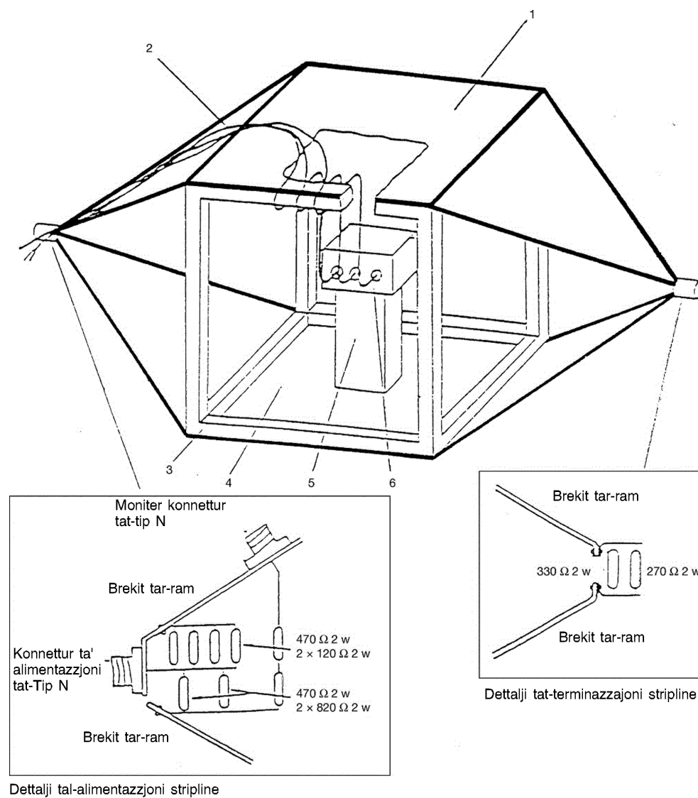
Figura 3 Ittestjar bl-istripline ta' 800 mm
