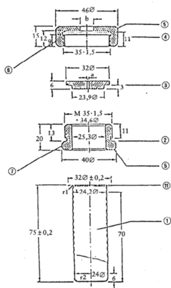
Fig. 1a Tubu ta' l-azzar u aċċessorji
