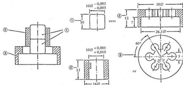
Fig 4d. Apparat tax-xokk għal sustanzi likwidi
