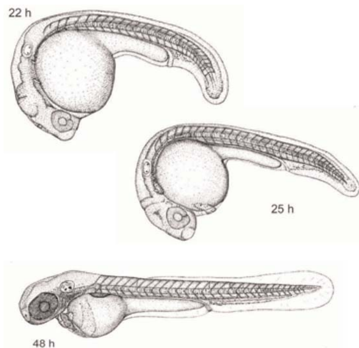
Grafika 1: Stadji magħżula tal-iżvilupp kmieni taż-żebra ( Danio rerio ): 0,2 — 1,75 siegħa wara l-fertilizzazzjoni (minn Kimmel et al. , 1995 (35)). Is-sekwenza taż-żmien mill-iżvilupp normali tista' tittiehed għad-djanjosi kemm tal-fertilizzazzjoni kif ukoll tal-vijabbiltà tal-bajd (ara l-paragrafu 26: Għażla tal-bajd fertilizzat).
