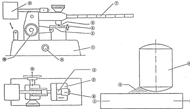
Fig 5a. Apparat ta'frizzjoni; elevazzjoni u veduta mill-ġenb
