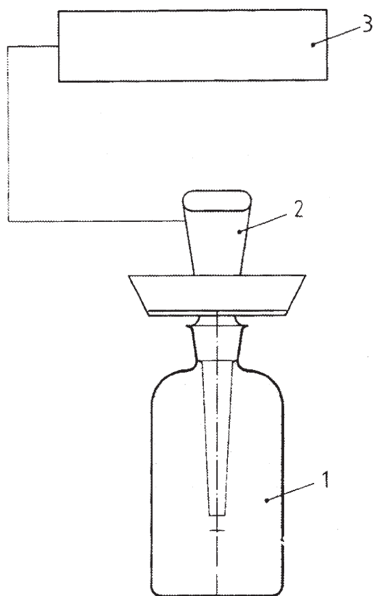
Fig. 2: Eżempju tal-unità tal-kejl, permezz ta' flixkun BOD
