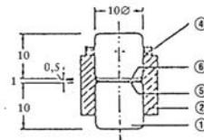
Fig 4d. Apparat tax-xokk għal sustanzi likwidi
