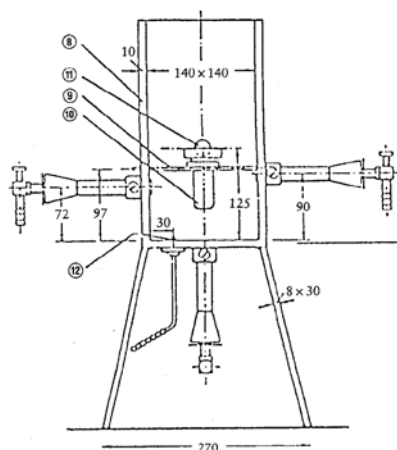
Fig. 1b Apparat ta' tishin u protettiv
