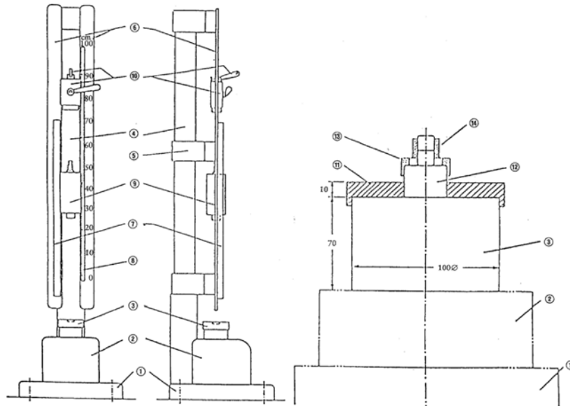
Fig 4b Martell li jaqa', il-parti t'isfel
