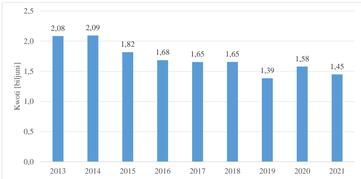
Illustrazzjoni 5. Eċċess tal-kwoti fl-EU ETS (2013-21).
