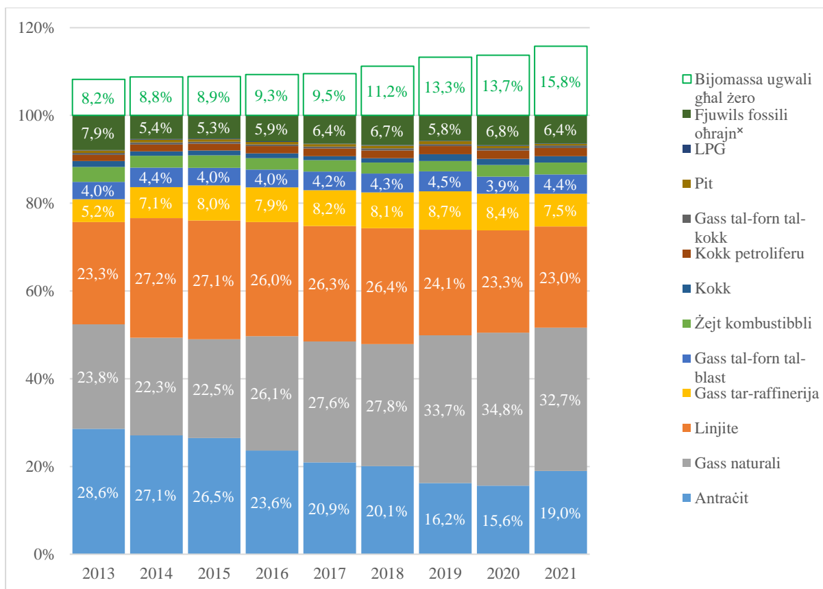
Illustrazzjoni 3. Emissjonijiet skont it-tip ta' fjuwil bħala ishma tal-emissjonijiet annwali tal-fjuwils fossili. Il-fjuwils fossili flimkien jammontaw għal 100 %, il-bijomassa tiżdied ma' dan. It-tikketti ma jidhrux jekk il-fjuwil qatt ma jaqbeż it-3 % tat-total, * = mhux kopert mill-fjuwils speċifikati l-oħrajn.
