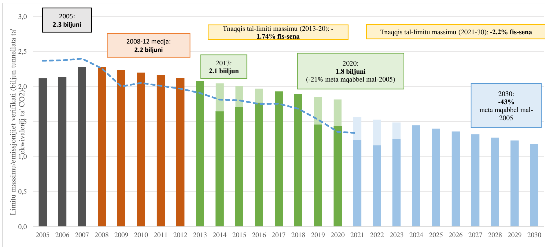
Illustrazzjoni 1. Limitu massimu tal-emissjonijiet stabbilit fl-EU ETS, meta mqabbel mal-emissjonijiet ivverifikati. Didaskalija: kolonni (limitu), kolonni çari fl-2014-16 (kwoti kkonċentrati fl-aħħar tal-perjodu fil-fażi 3), kolonni çari mill-2019 (għotjiet tal-kwoti għar-Riżerva tal-Istabbiltà tas-Suq), linja miksura (emissjonijiet ivverifikati).
