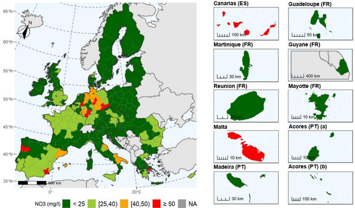
Illustrazzjoni 2: Il-koncentrazzjonijiet medji annwali tan-nitrati fl-ilma ta' taħt l-art fil-livell tan-NUTS 2 għall-perjodu ta' rapportar 2016-2019
