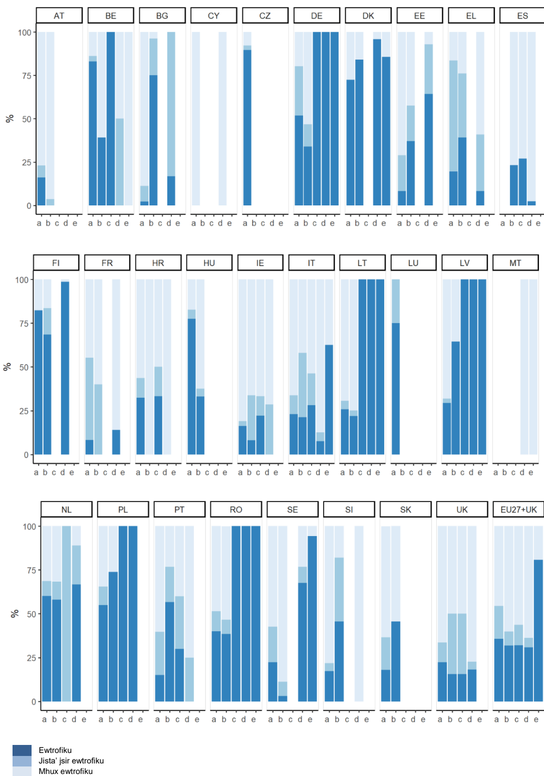
Illustrazzjoni 3: Dijagramma tal-frekwenza tal-istatus trofiku tax-xmajjar (a), tal-lagi (b), tal-ilmijiet tranżizzjonali (c), tal-ilmijiet kostali (d) u tal-ilmijiet marittimi (e) fil-perjodu ta' rapportar 2016-2019.
