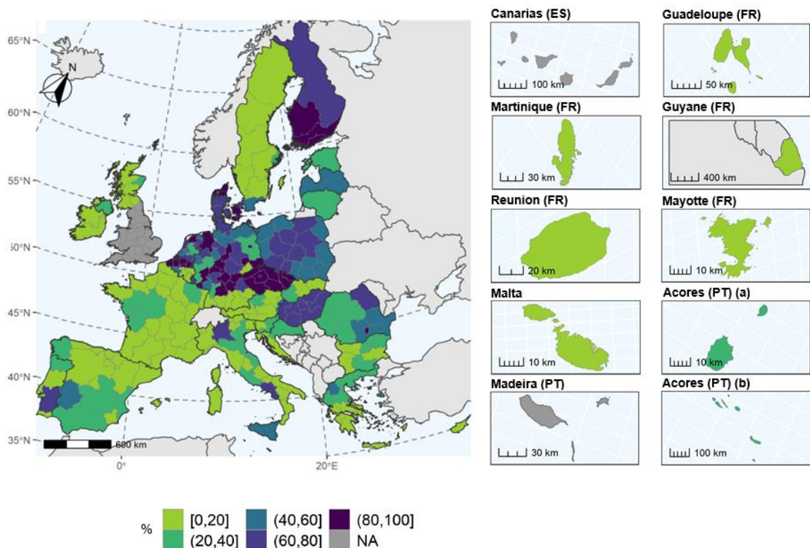
Illustrazzjoni 4: Il-percentwal ta' stazzjonijiet tal-ilmijiet tal-wiċċ (il-kategoriji kollha) fi status ewtrofikku fil-livell tan-NUTS 2, għall-perjodu ta' rapportar 2016-2019
