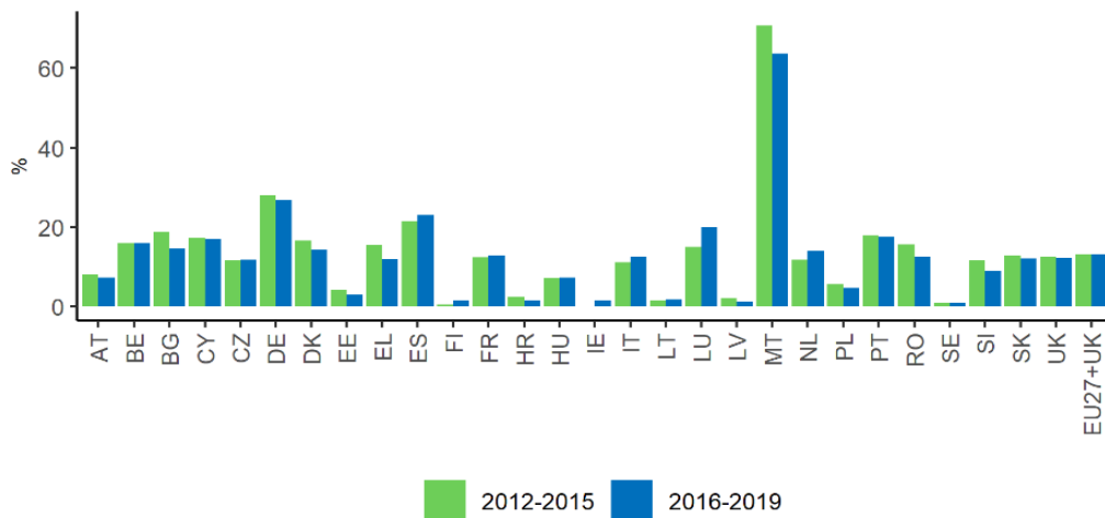
Illustrazzjoni 1: perċentwal ta' stazzjon tal-ilma ta' taħt l-art li jaqbeż il-50 mg nitrati għal kull litru.
