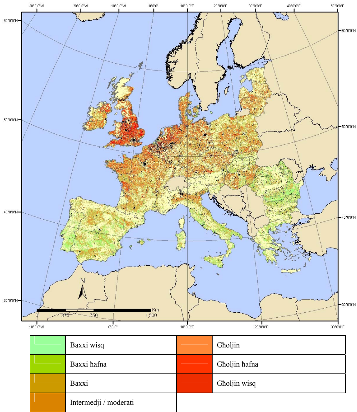
Figura 5: Theddidiet potenzjali għall-bijodiversità tal-ħamrija.
