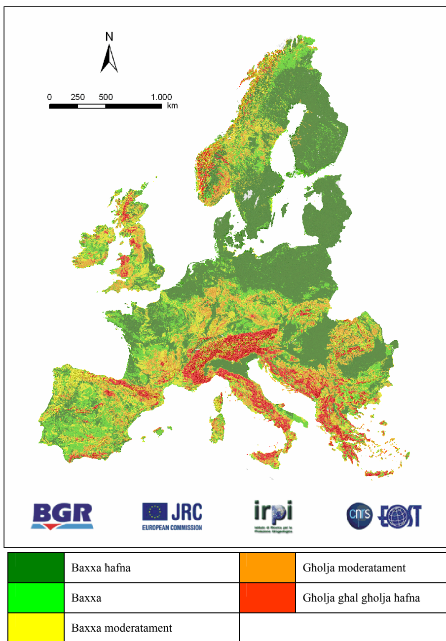
Figura 6: Suxxettibbiltà għall-uqigh tal-art fl-UE u f'pajjiżi girien (mappa preliminari) 38 .
