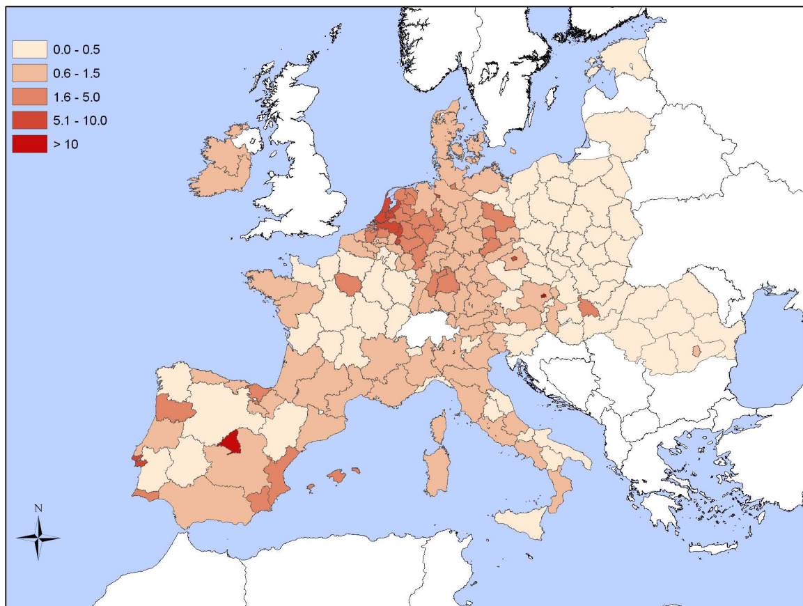
Figura 2: Telfiet potenzjali ta' rendiment ta' qamh (%) f'19-il pajjiż tal-UE (1990-2006).
