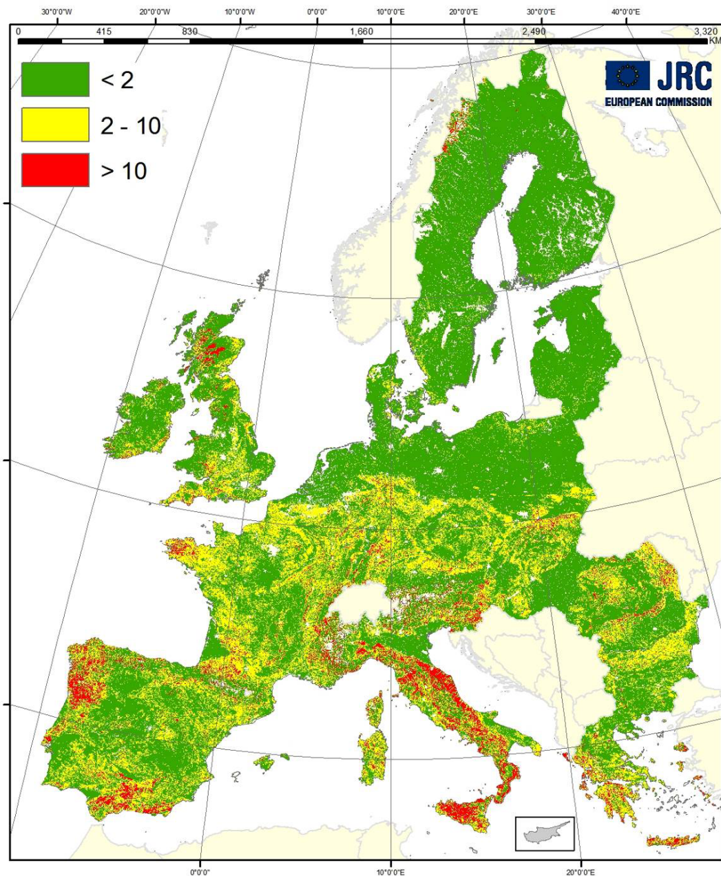
Figura 3: Erożjoni tal-ħamrija mill-ilma fl-UE (t/ha/y).
