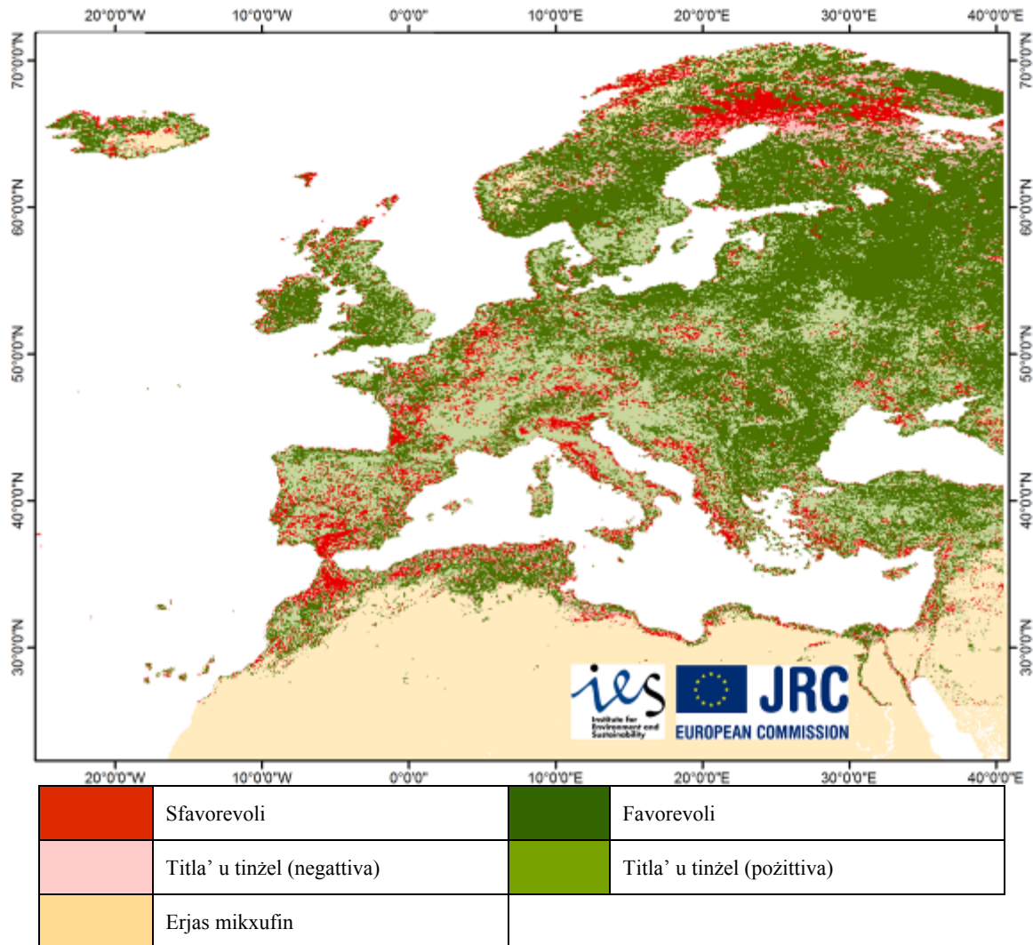
Figura 4: Evoluzzjoni tal-produttività primarja netta (1982-2006).
