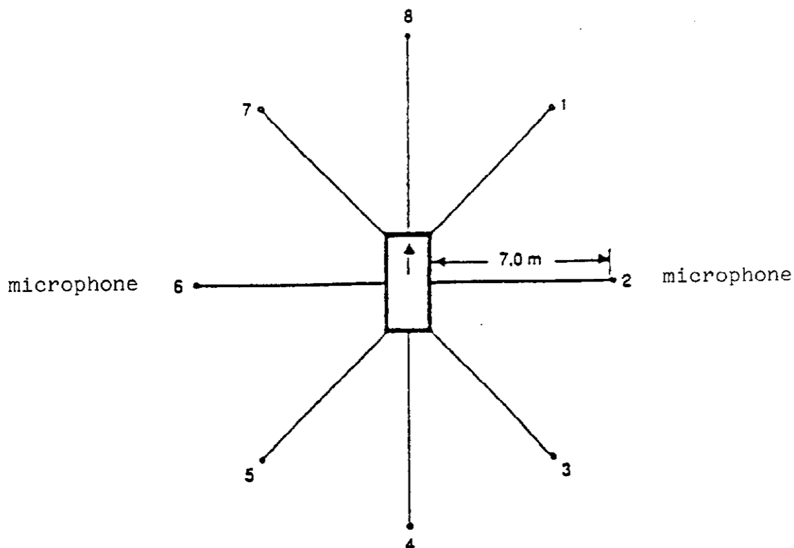
Figura 1: Il-pożizzjonijiet tal-mikrofonu għall-kejl tal-ħoss tal-arja kkompessata
