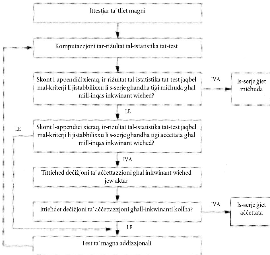
Figura 2.1 Skematika tal-ittestjar tal-konformità tal-produzzjoni
