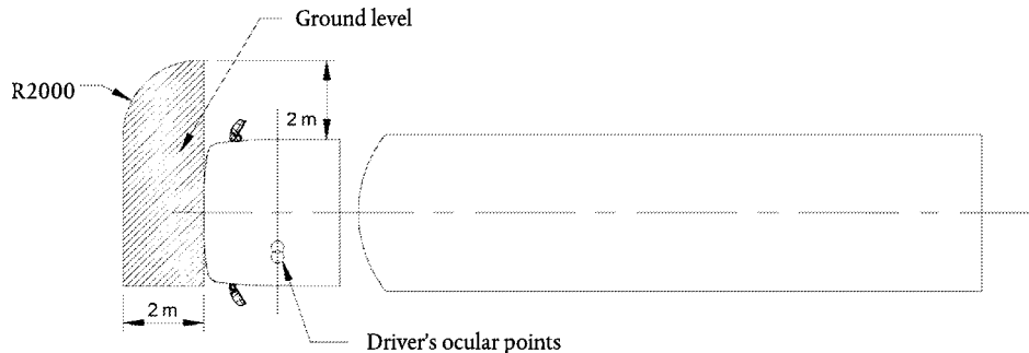
11 attēls: VI klases priekšējā spoguļa redzamības lauks
