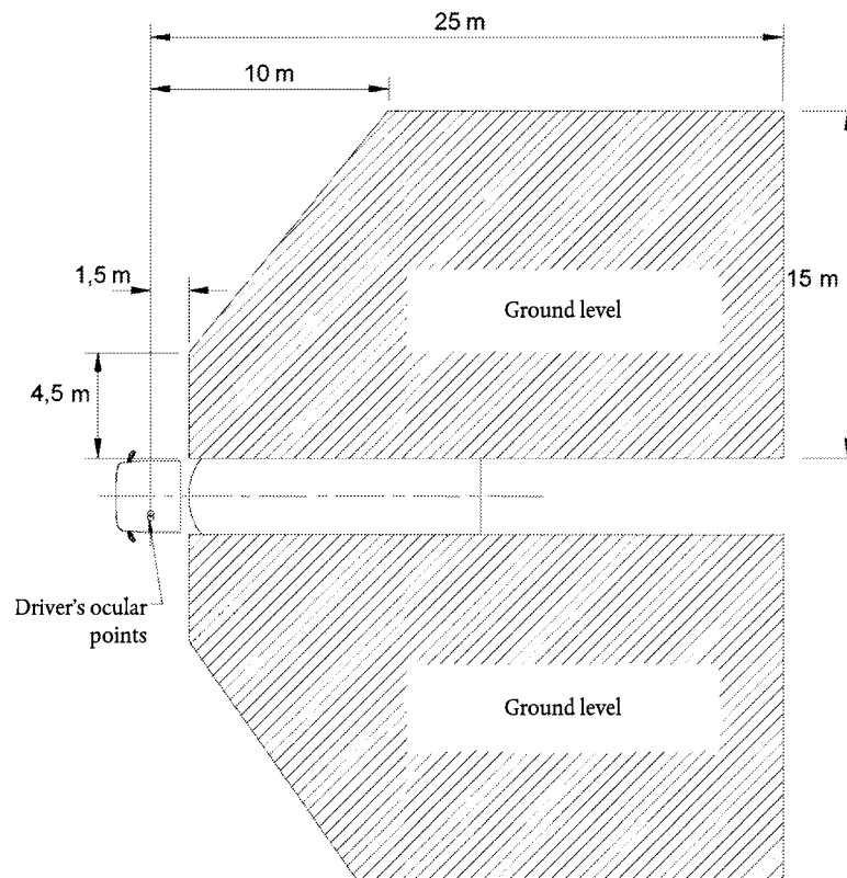
9. attēls: IV klases platleņķa spoguļu redzamības lauks
