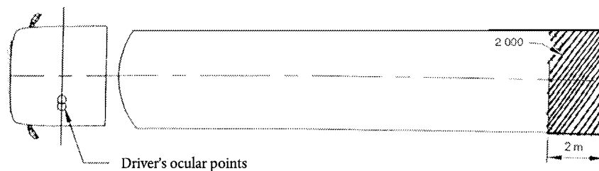
12. attēls: Aizmugurējo netiešās redzamības ierīču redzamības lauks
