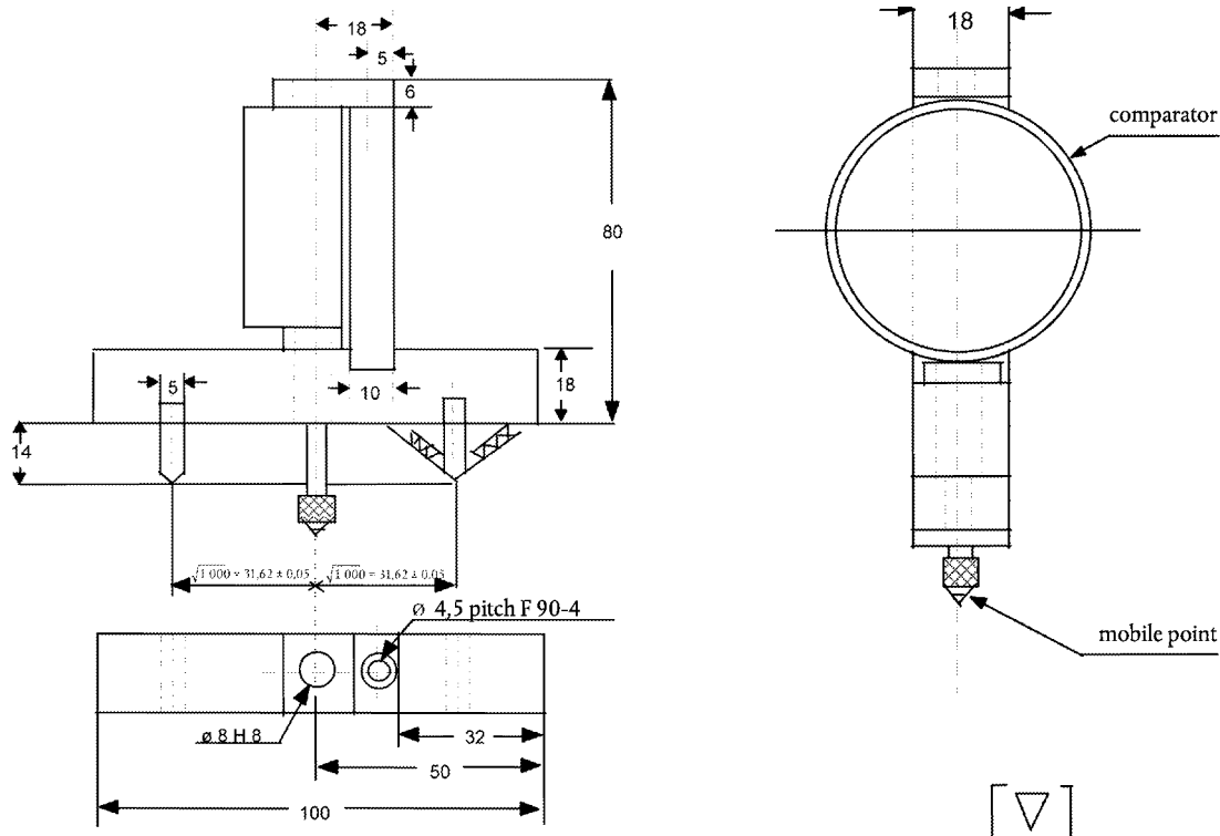
3. attēls: sferometrs
