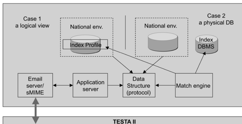
2 paveikslas. Programos topologijos apžvalga
