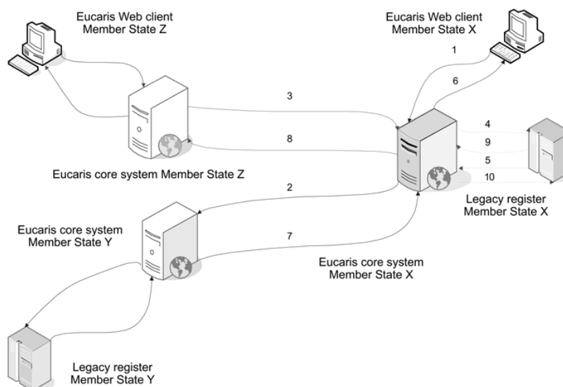
5 paveikslas. Registravimui skirti pranešimų tipai
