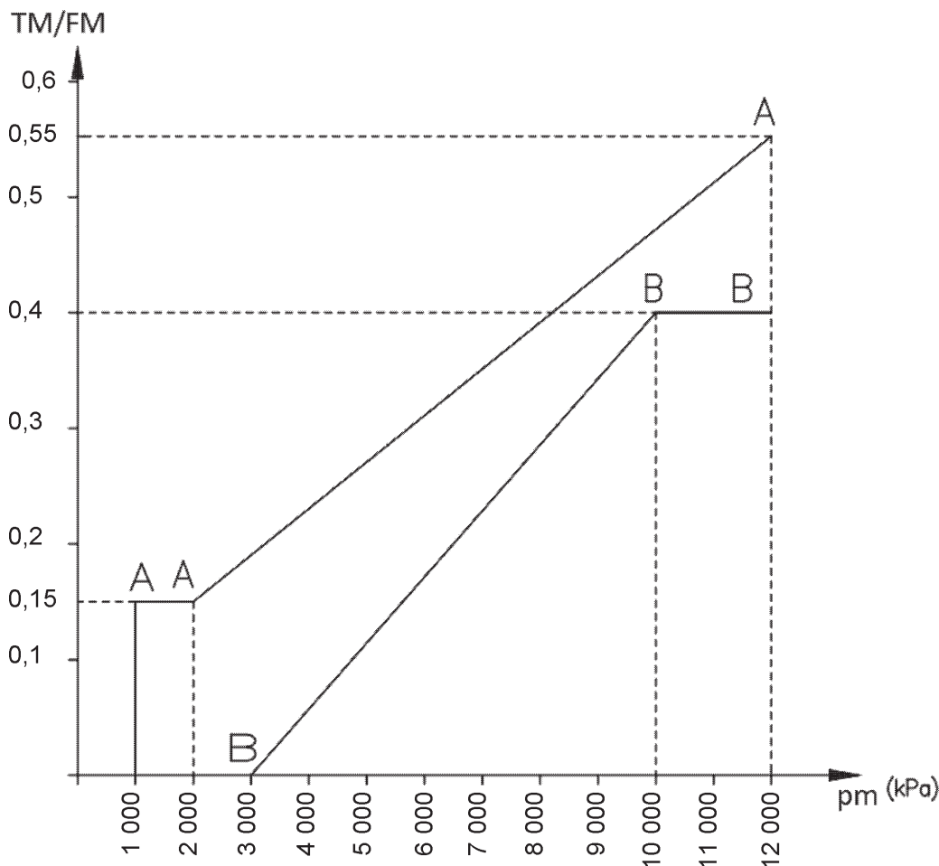
Stabdymo greičio (TM/FM) ir sukabintuvo slėgio (pm) santykis
