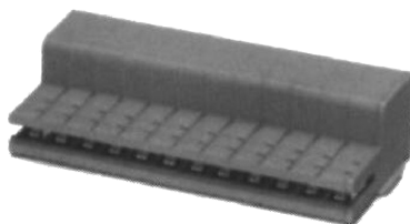
8 pav. Vienpusis jungiamasis elementas tiesiogiai prijungiamas prie spausdintinės plokštės
