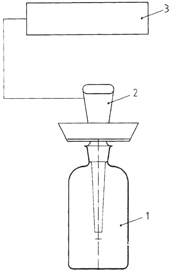
2 pav. Su BDS buteliu naudojamo matavimo prietaiso pavyzdys
