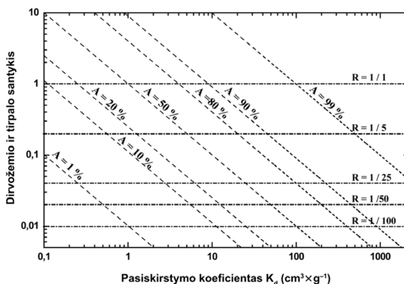
1 pav., Dirvožemio/tirpalo santykio ir K_d sąryšis esant įvairioms adsorbuotos medžiagos procentinėms dalims
