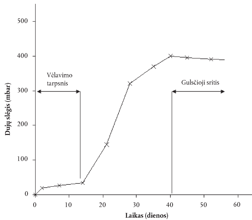
Skaidymo kreivės pavyzdys (suminis neto slėgio padidėjimas)
