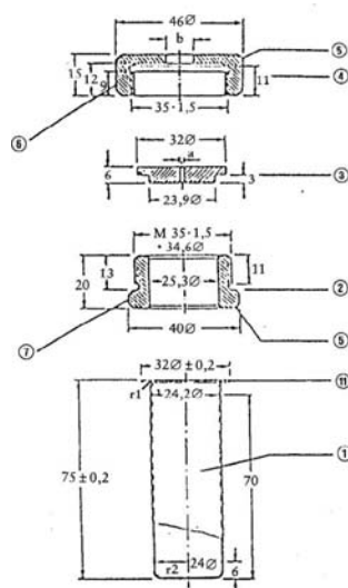
1a pav. Plieninis vamzdis s ir priedai
