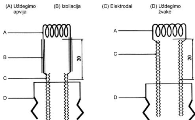
3 paveikslas Uždegimo sistema
