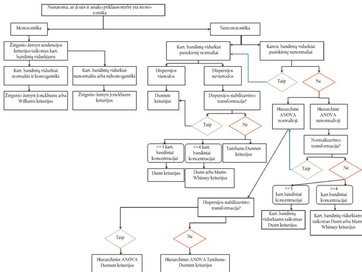
Statistinei analizei skirta srautinė sprendimų diagrama
