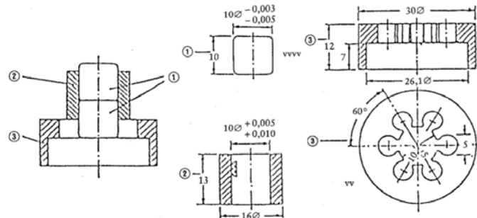
4c pav. Smūgiavimo įtaisas miltelių arba pastos pavidalo medžiagoms
