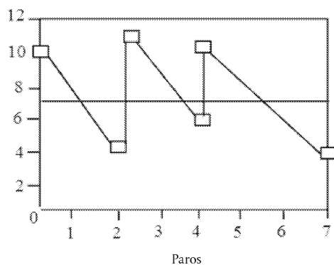
Laikinio svertinio vidurkio pavyzdys
