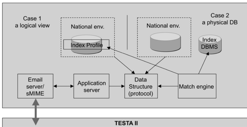
Figura 2: Quadro della topologia dell'applicazione
