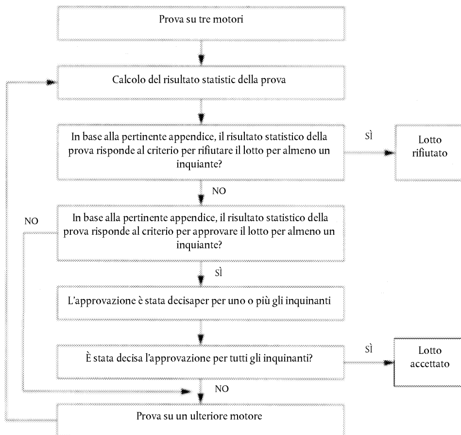
Figura 2.1 Schema della prova di conformità della produzione
