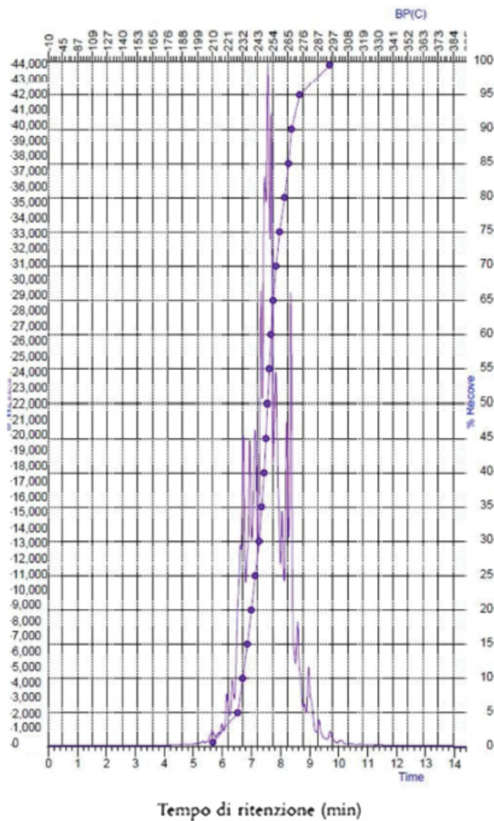
SIMDIS ASTM D 2887 extended, correlazione con ASTM D 86
