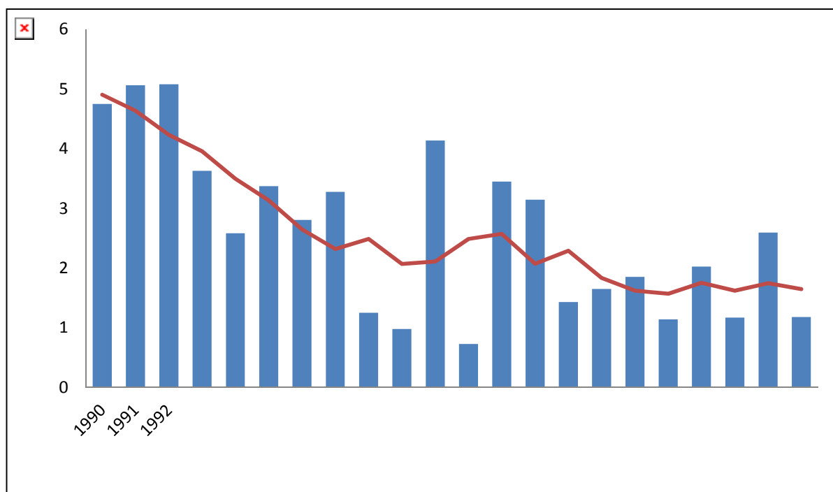
Figura 7: scontri ferroviari e deragliamenti mortali per miliardo di treni-chilometro
