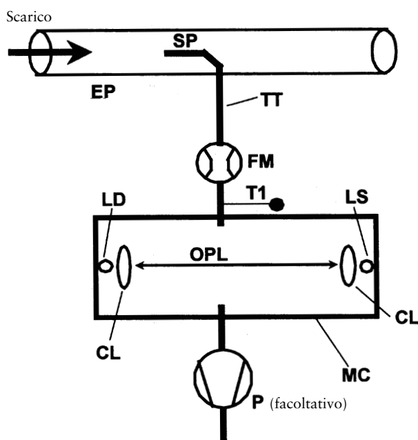
Opacimetro a flusso parziale
